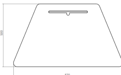
Ripiano per composizione ottagonale
